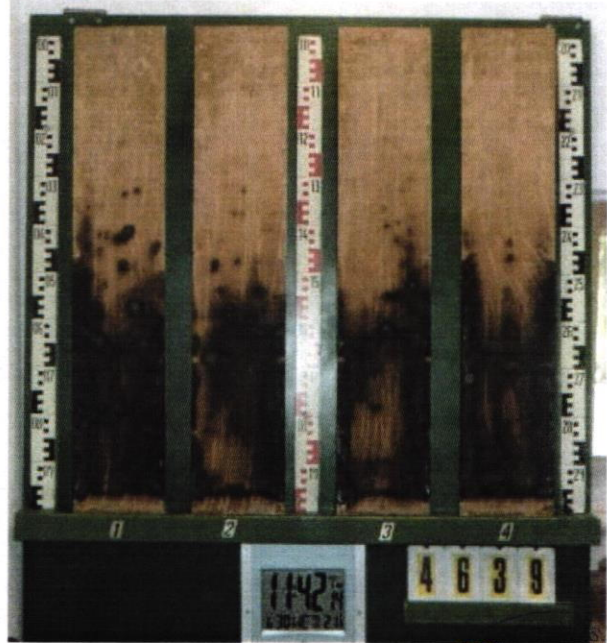
Restlänge Spanplatte
