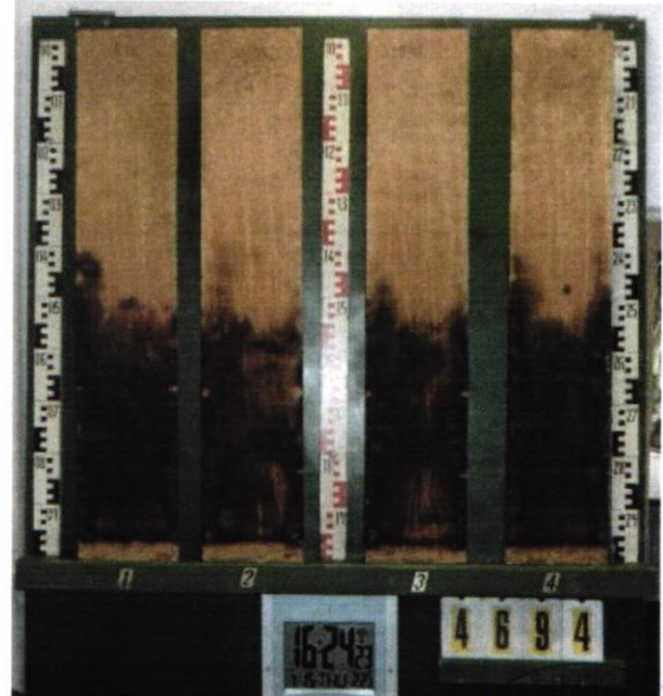
Restlänge Spanplatte
