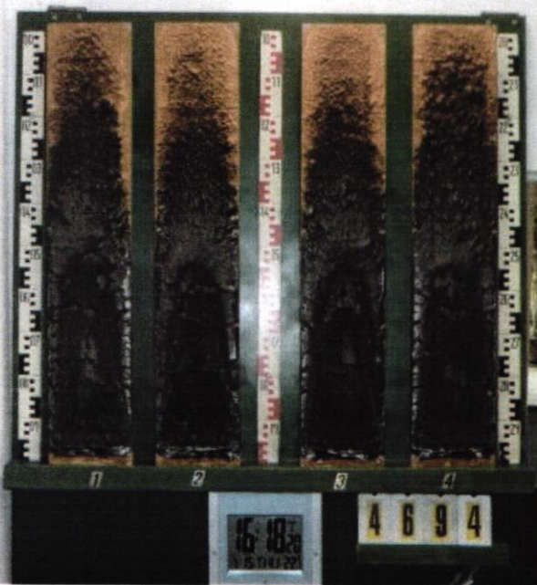
Restlänge Dämmschichtbildner
