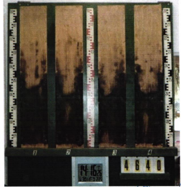
Restlänge Spanplatte
