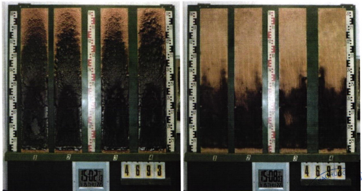
Restlänge Dämmschichtbildner
